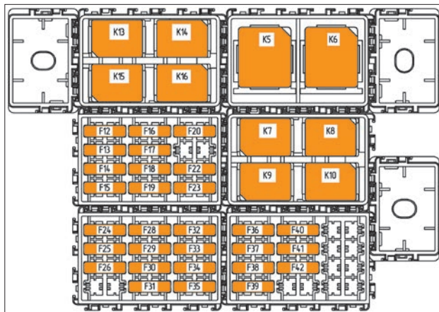
Рис. 48. Схема монтажного блока в салоне с нумерацией предохранителей и реле
