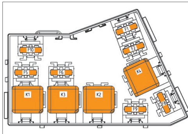
Рис. 49. Схема монтажного блока в моторном отсеке с нумерацией предохранителей и реле
