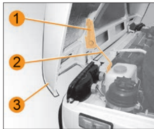
Рис. 7. Упор капота
